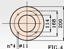
n°4 Ø11
